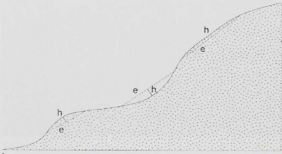
Abb. 4 Schätzung der Wölbungsstärke (nach FINNERN et al. 1996, 61 Abb. 6).
