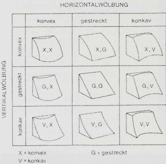
Abb. 3 Schema zur Kennzeichnung der Wölbungsrichtung (vertikal, horizontal) und Wölbungstendenzen (konvex, gestreckt, konkav) (aus FINNERN et al. 1996, 63 Abb.7).
