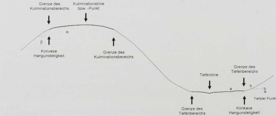
Abb. 5 Skizze zur Definition von Kulmiations- und Tiefenbereich (nach FINNERN et al. 1996, 65 Abb. 8; 66 Abb. 9).
